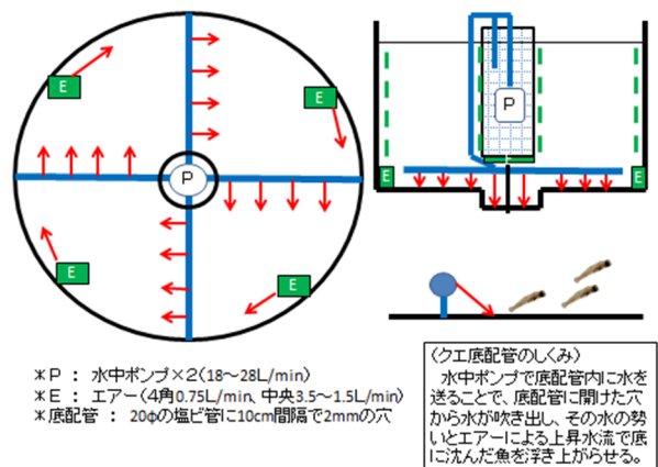
図2 クエの底配管図
