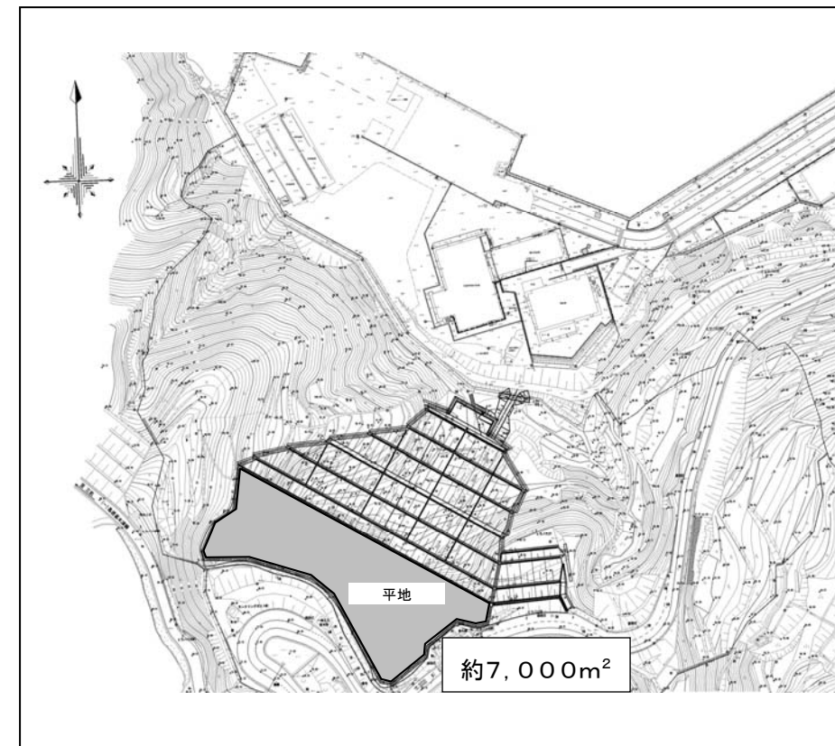
作業スペース①詳細図
