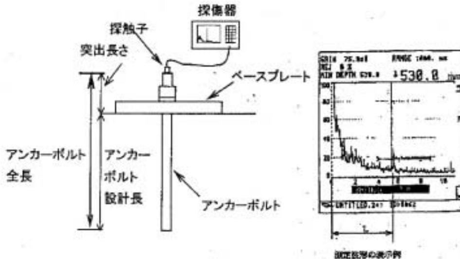
アンカーボルト長さの測定の例
