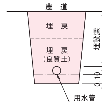
用水路工（パイプライン工）
