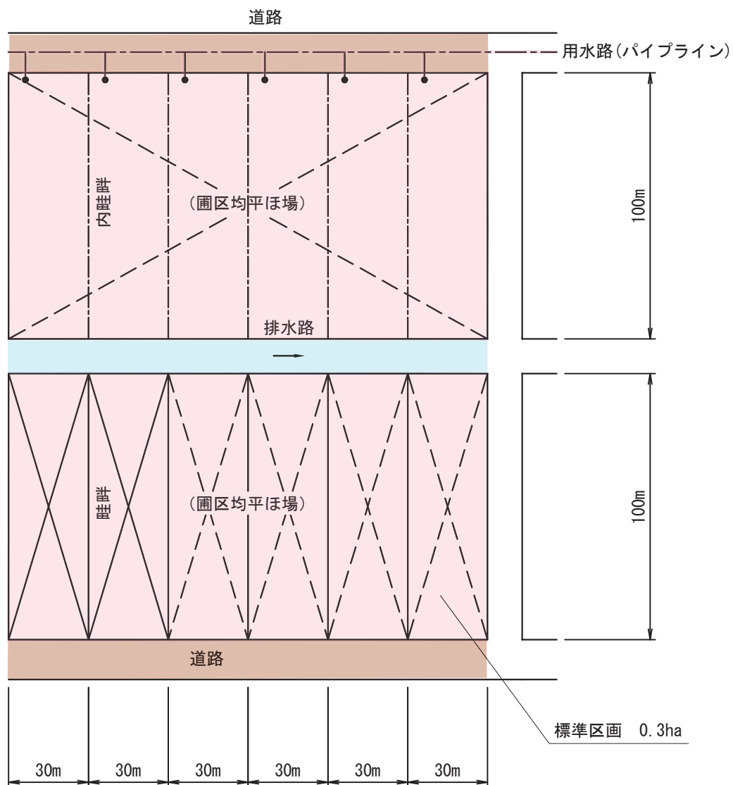
区画整理工（標準区画割図）
