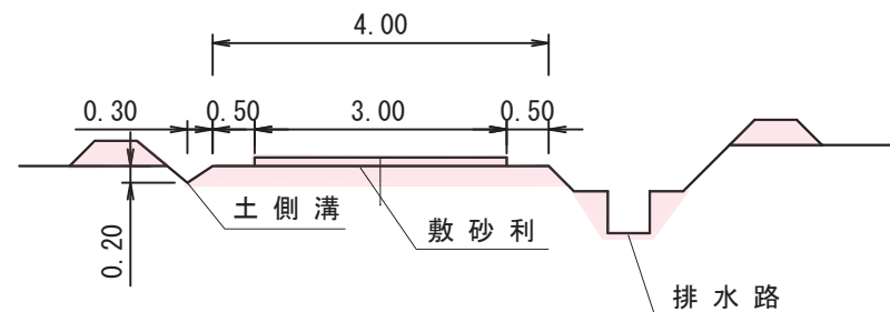
道路工（支線B道路）
