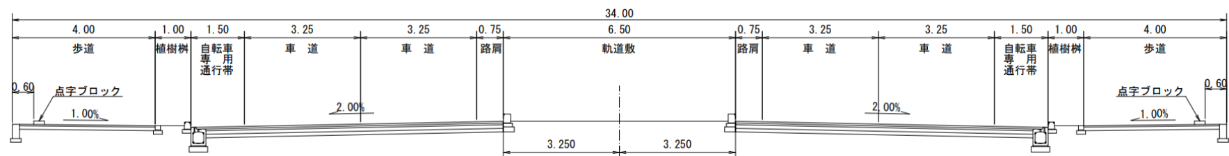
標準断面図
