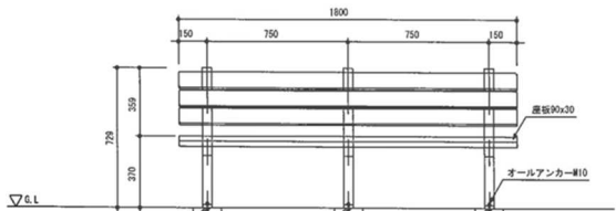
正面図
