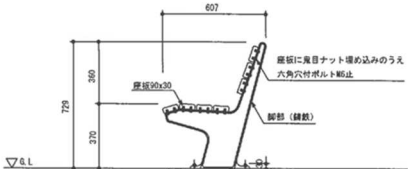
側面図
