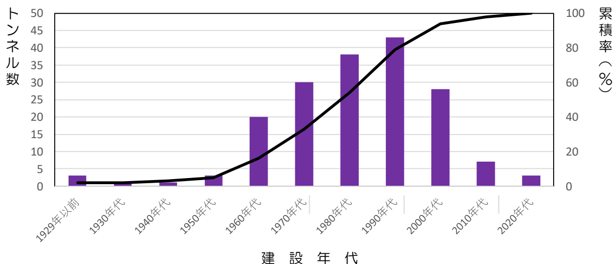
図2 建設年代別のトンネル数分布
