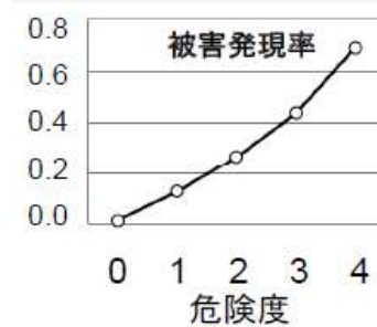
図 2.6-3 2004 年中越地震における検証結果（神谷（2013））
