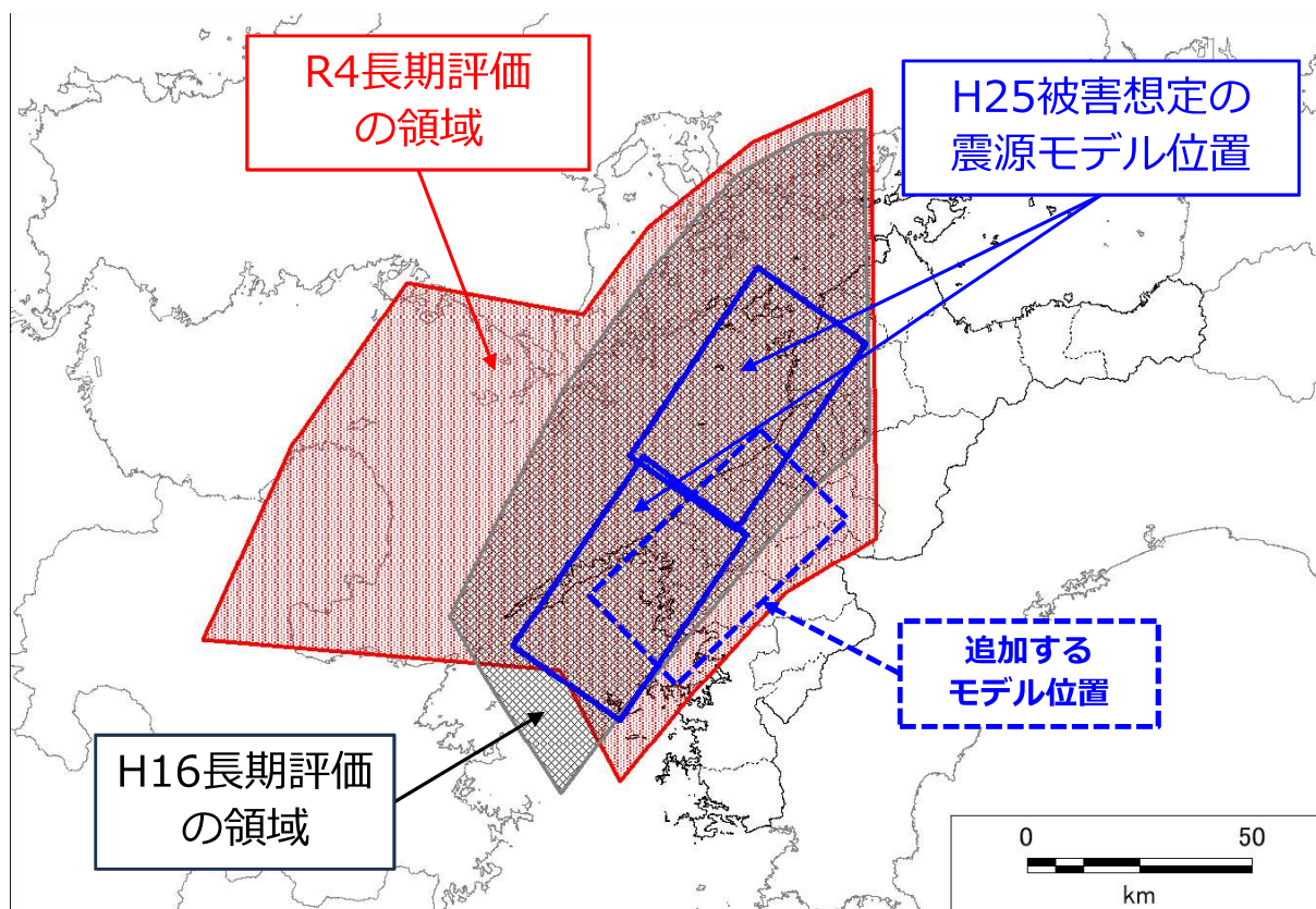
図 2.3-9 安芸灘～伊予灘～豊後水道のプレート内地震の震源領域
