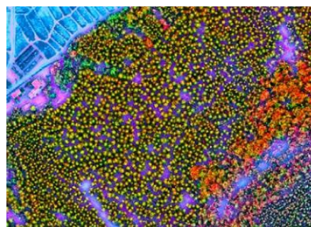
林相解析図
