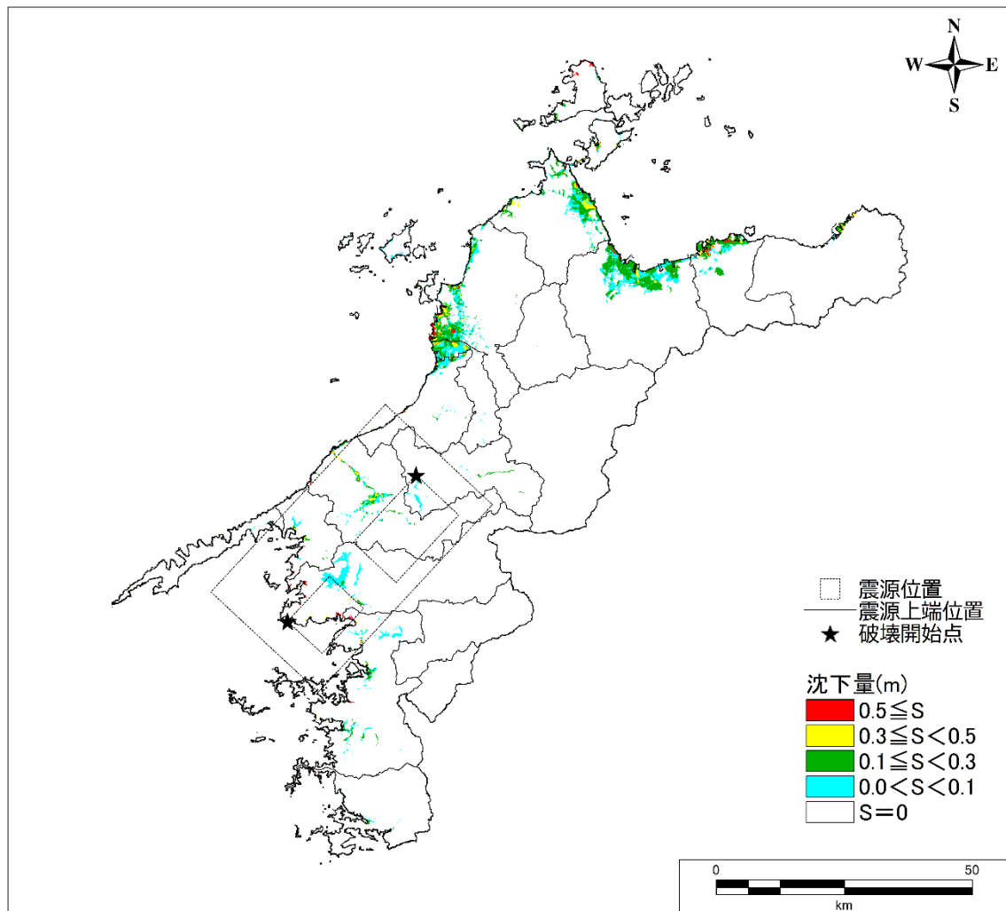
②” 安芸灘～伊予灘～豊後水道のプレート内の地震（モデルC）の沈下量分布
