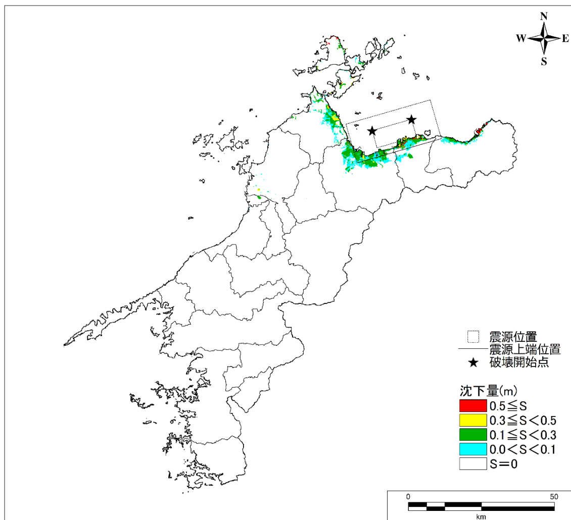
④中央構造線断層帯（石鎚山脈北縁区間）の沈下量分布
