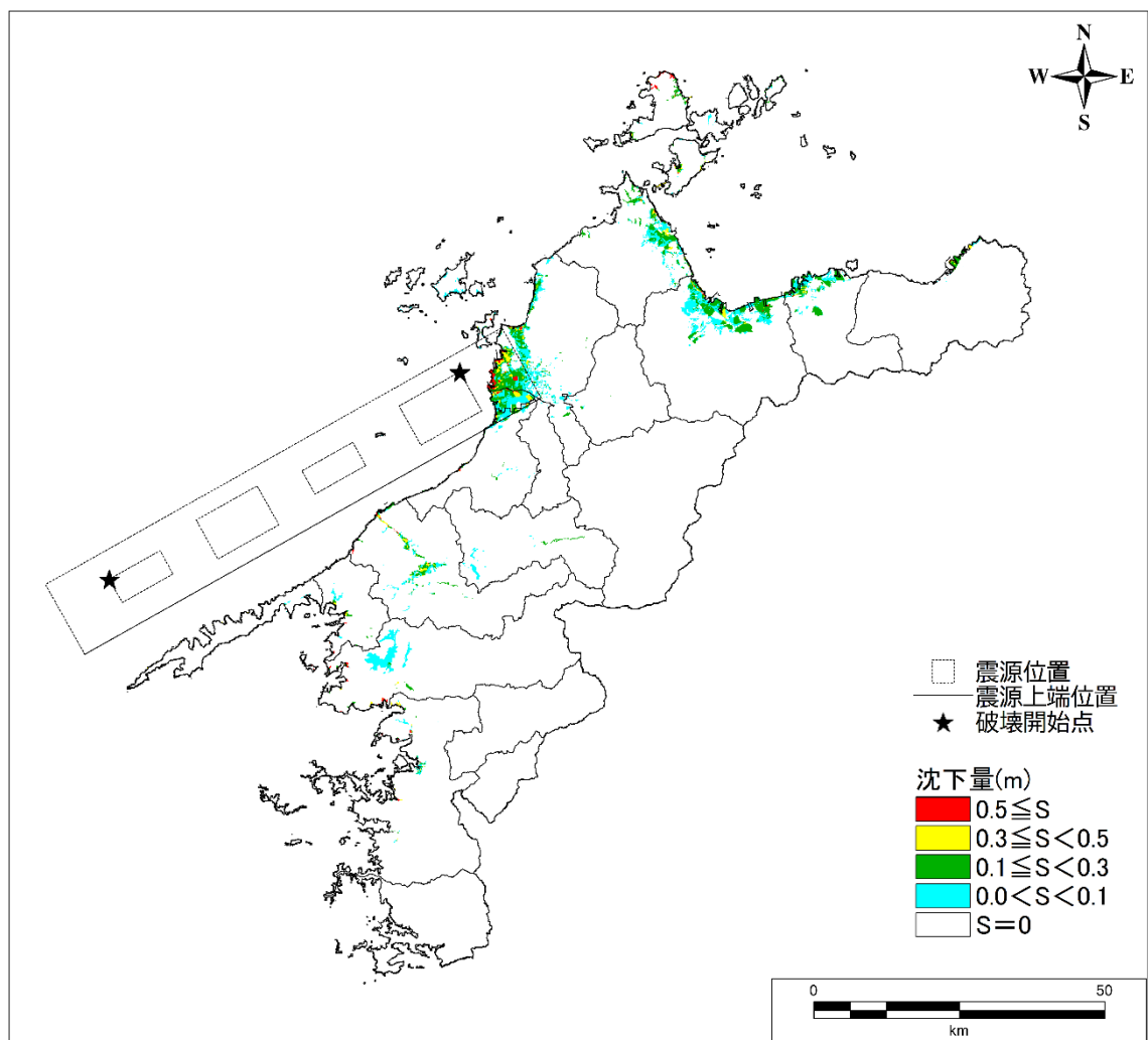
⑥中央構造線断層帯（伊予灘区間）の沈下量分布
