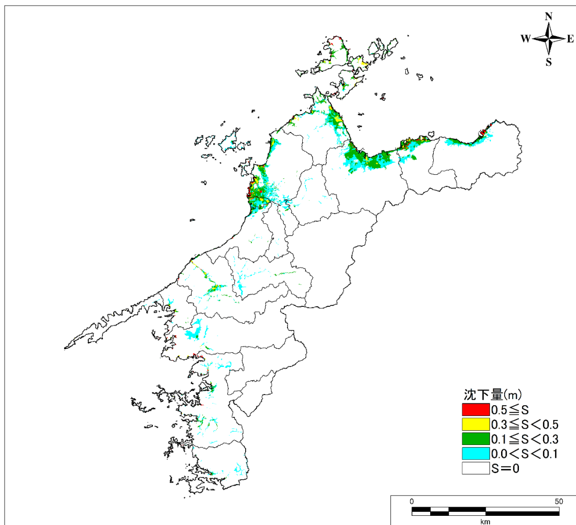
①南海トラフ巨大地震の沈下量分布
