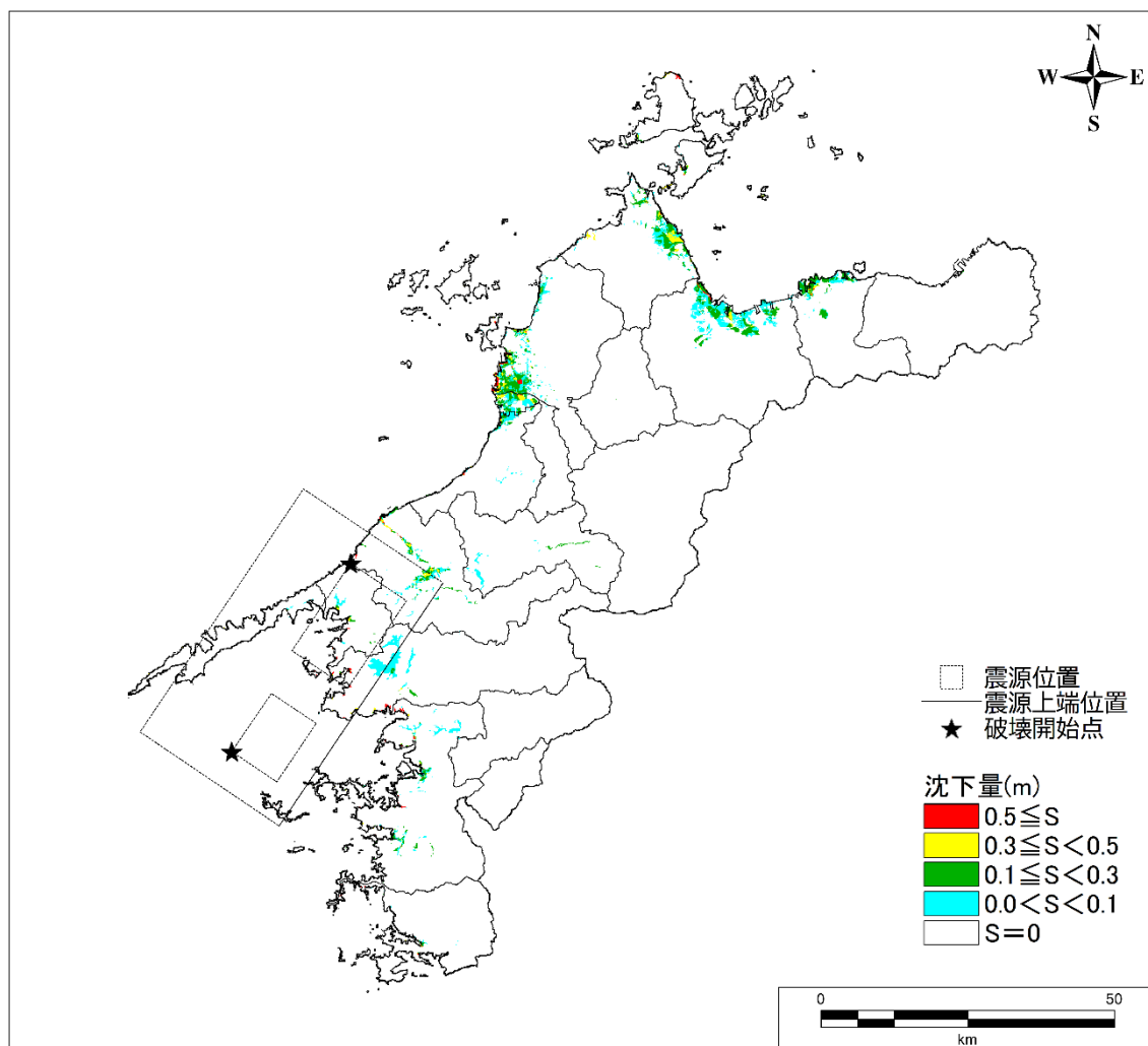
②' 安芸灘～伊予灘～豊後水道のプレート内の地震（モデル B）の沈下量分布
