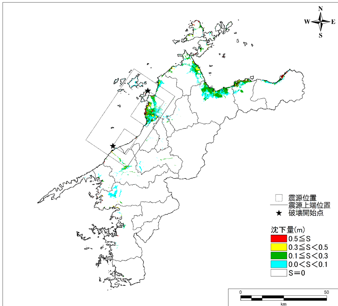
②安芸灘～伊予灘～豊後水道のプレート内の地震（モデル A）の沈下量分布
