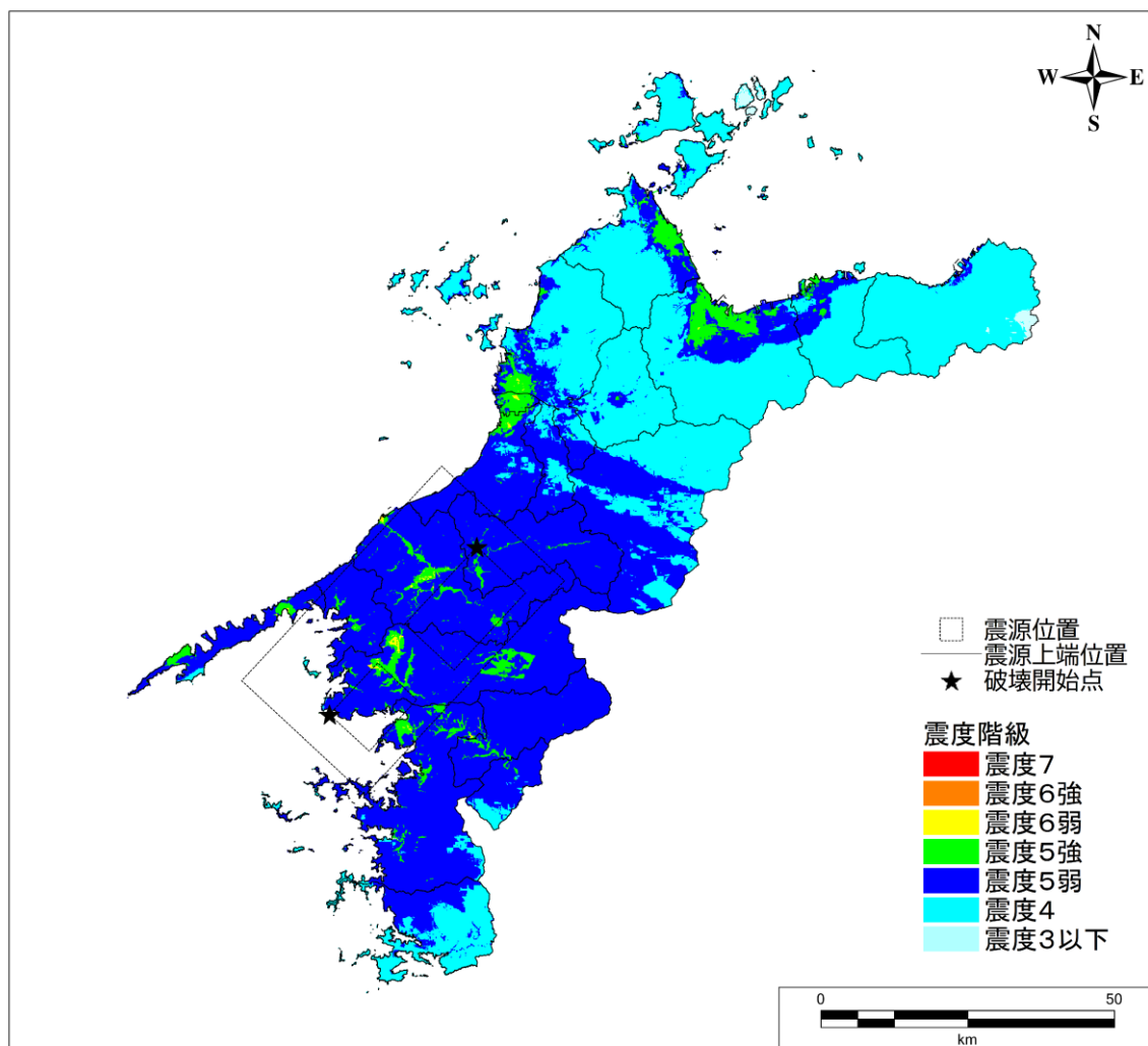
②” 安芸灘～伊予灘～豊後水道のプレート内の地震（モデルC）の震度分布
