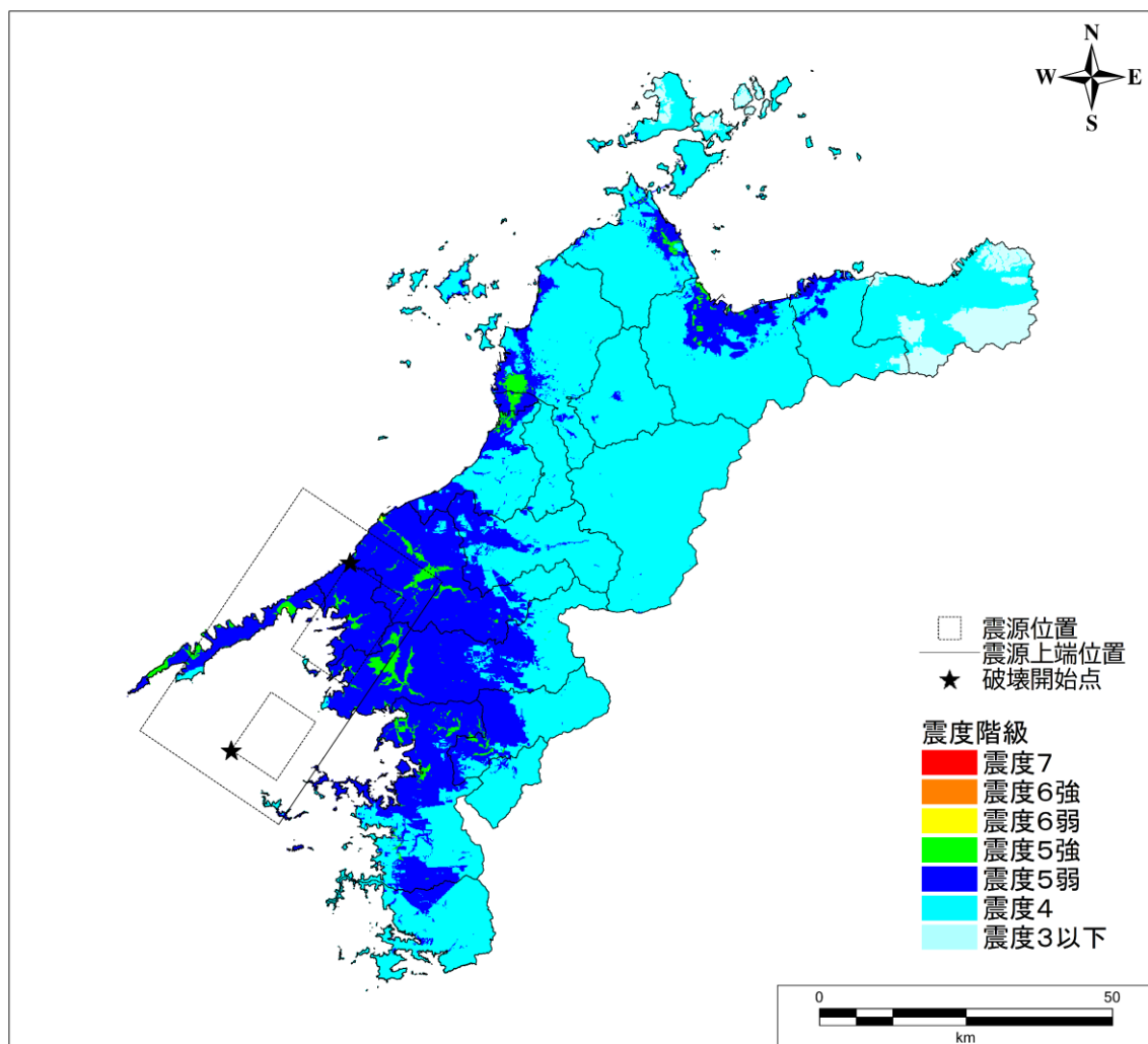
②' 安芸灘～伊予灘～豊後水道のプレート内の地震（モデル B）の震度分布
