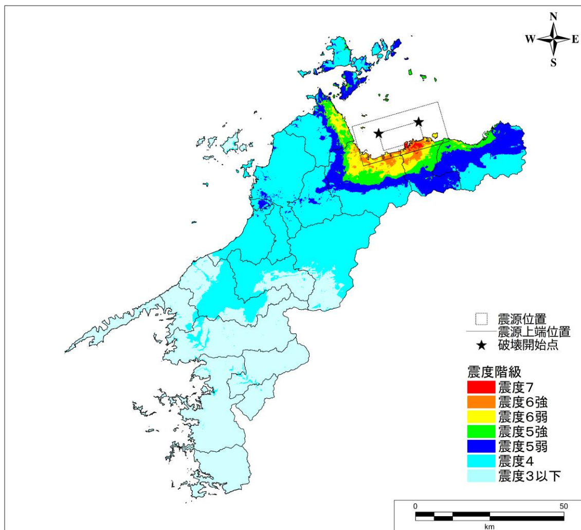
④中央構造線断層帯（石鎚山脈北縁区間）の震度分布
