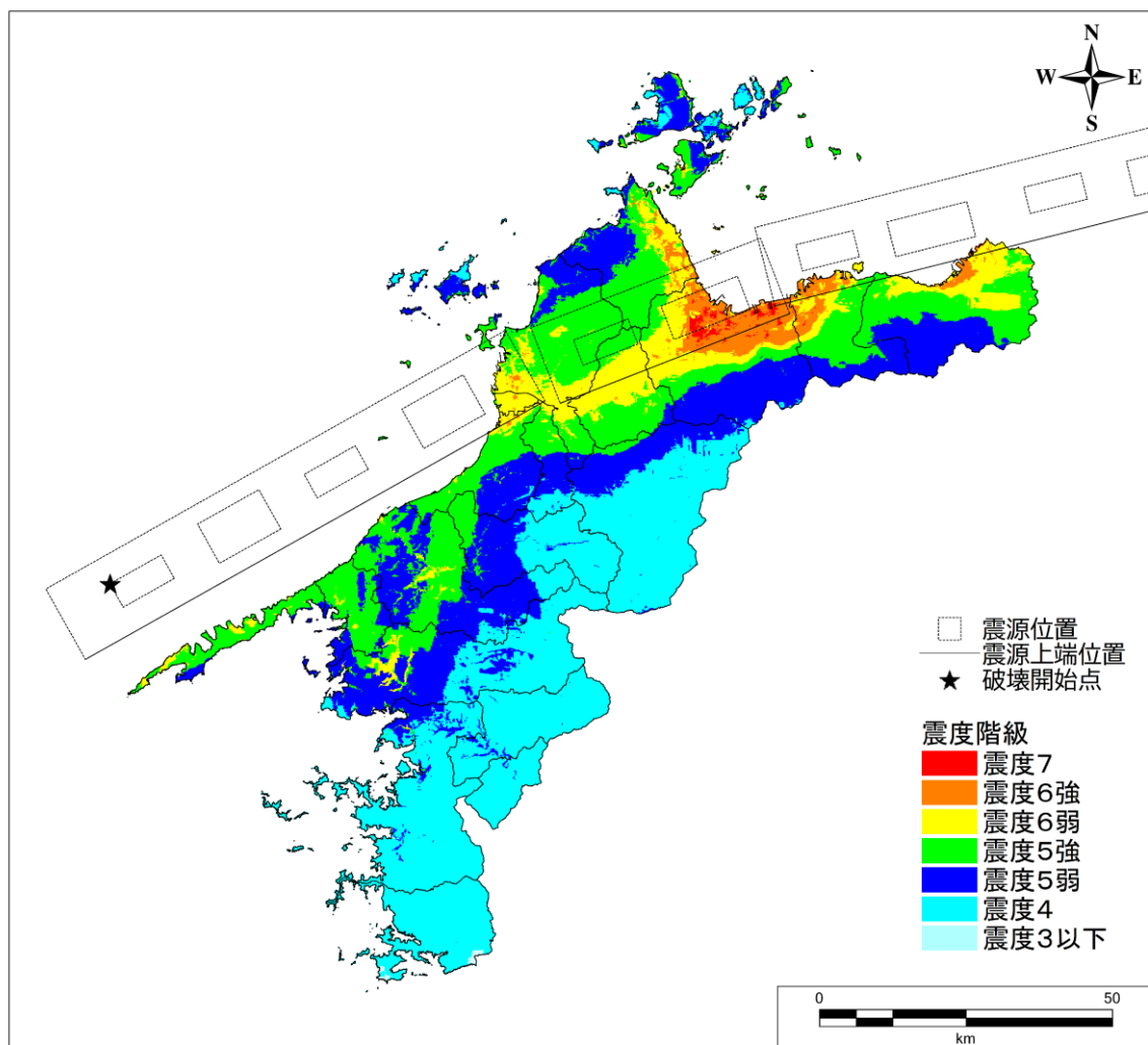
⑧中央構造線断層帯（3区間連動）の震度分布
