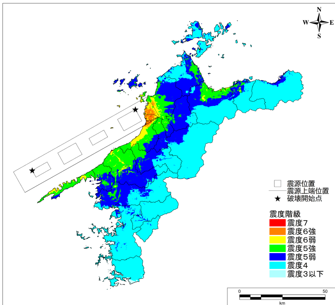
⑥中央構造線断層帯（伊予灘区間）の震度分布
