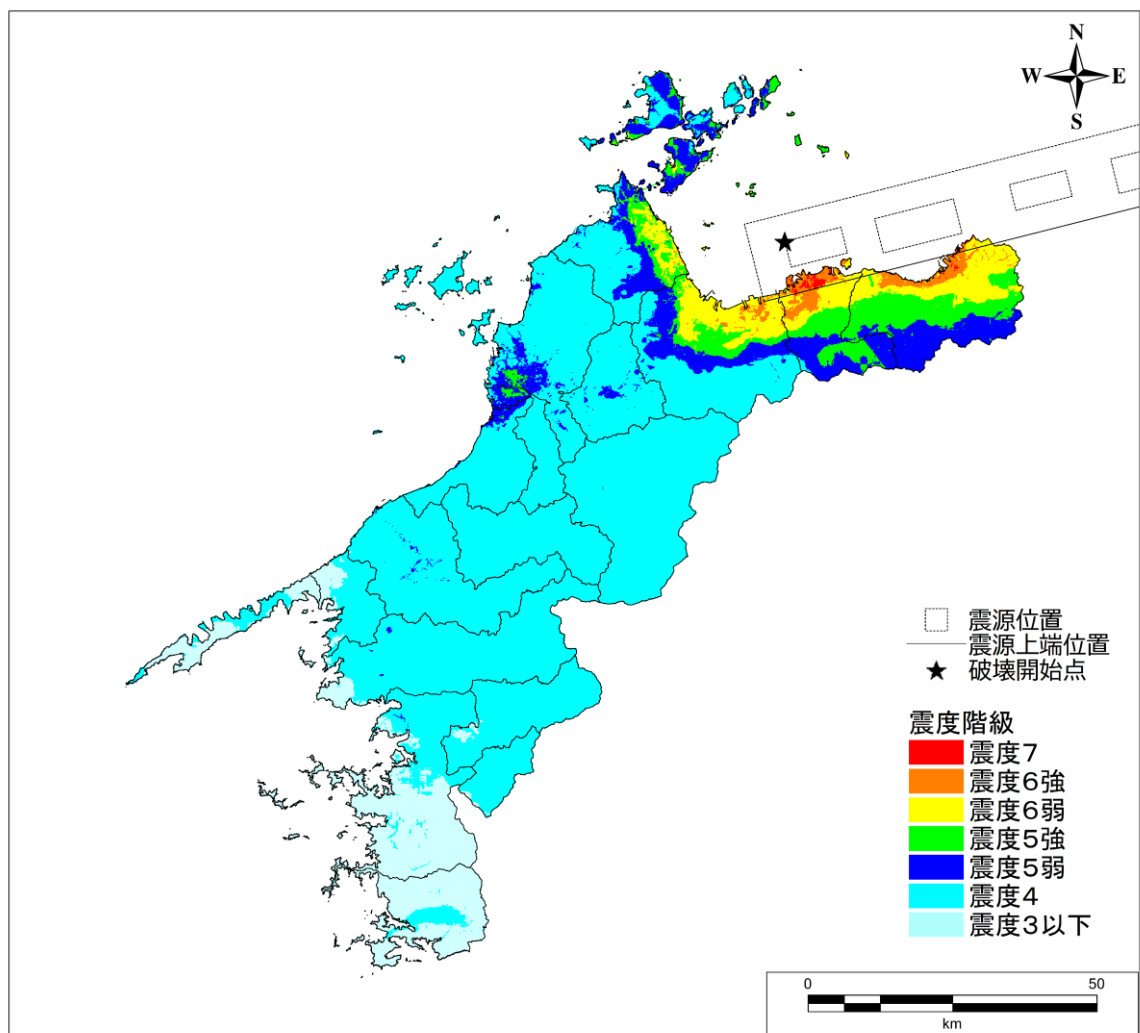
③中央構造線断層帯（讃岐山脈南縁西部区間）の震度分布
