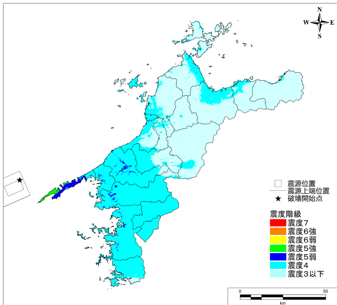
⑦中央構造線断層帯（豊予海峡-由布院区間）の震度分布
