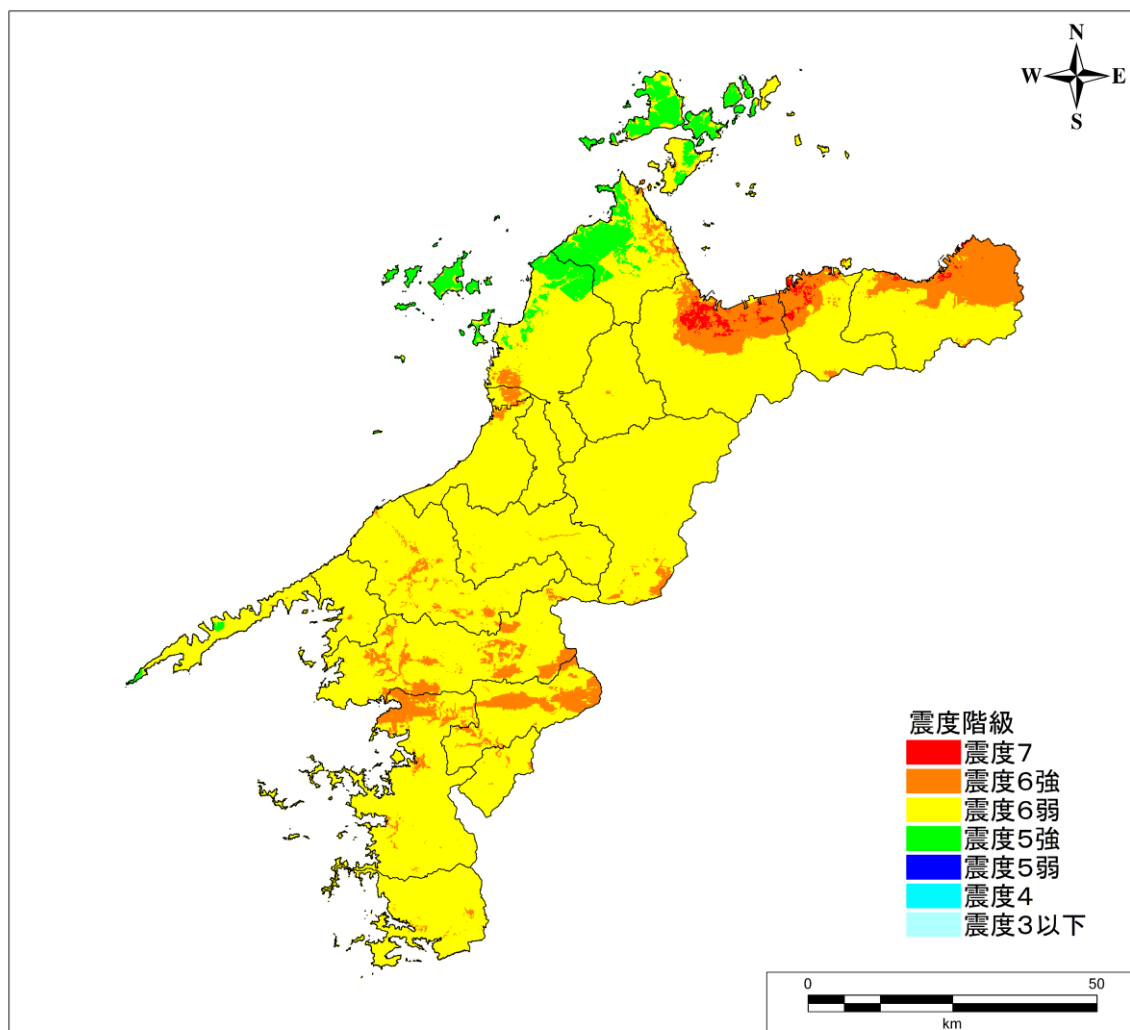
①南海トラフ巨大地震の震度分布
