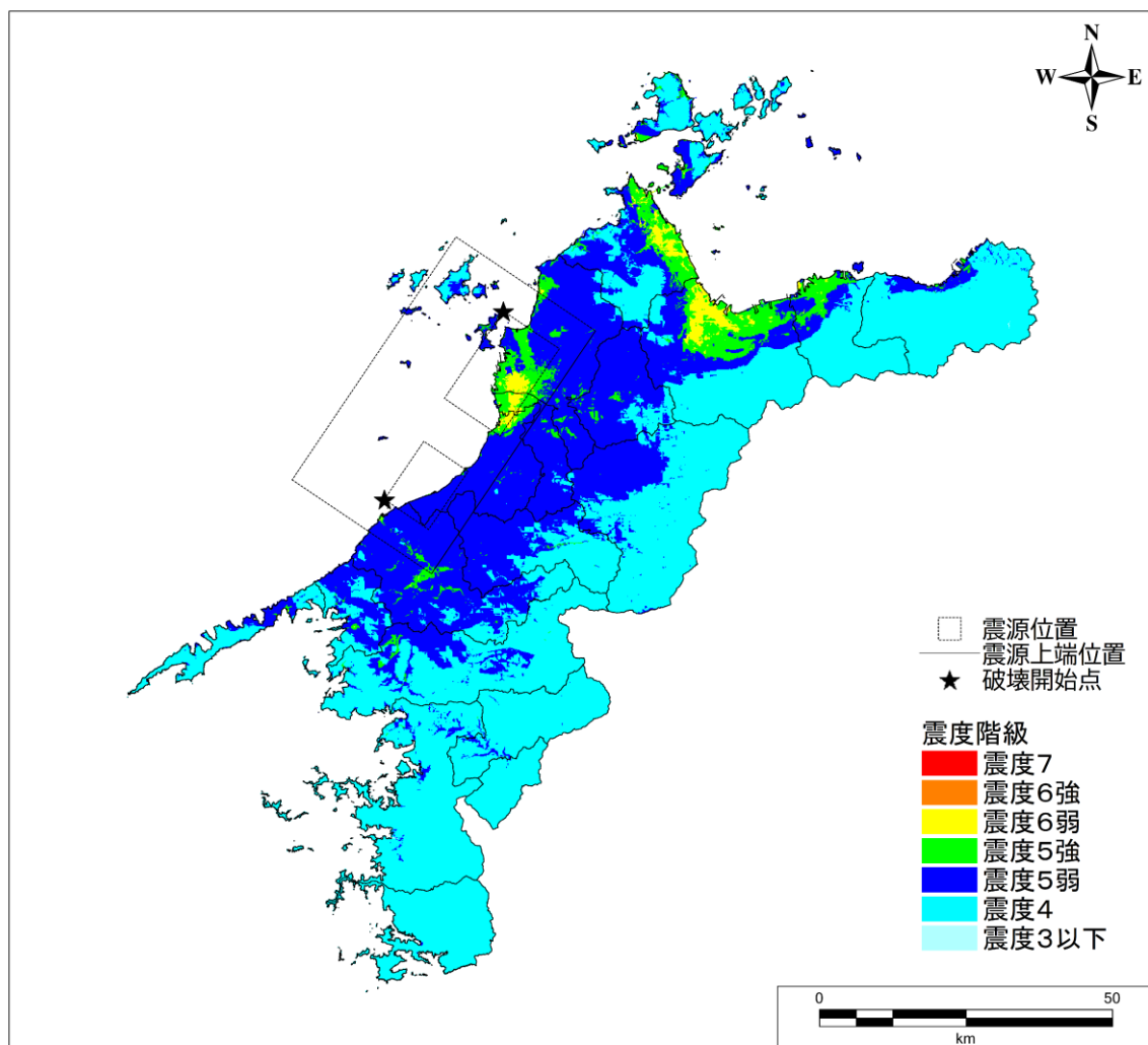
②安芸灘～伊予灘～豊後水道のプレート内の地震（モデル A）の震度分布
