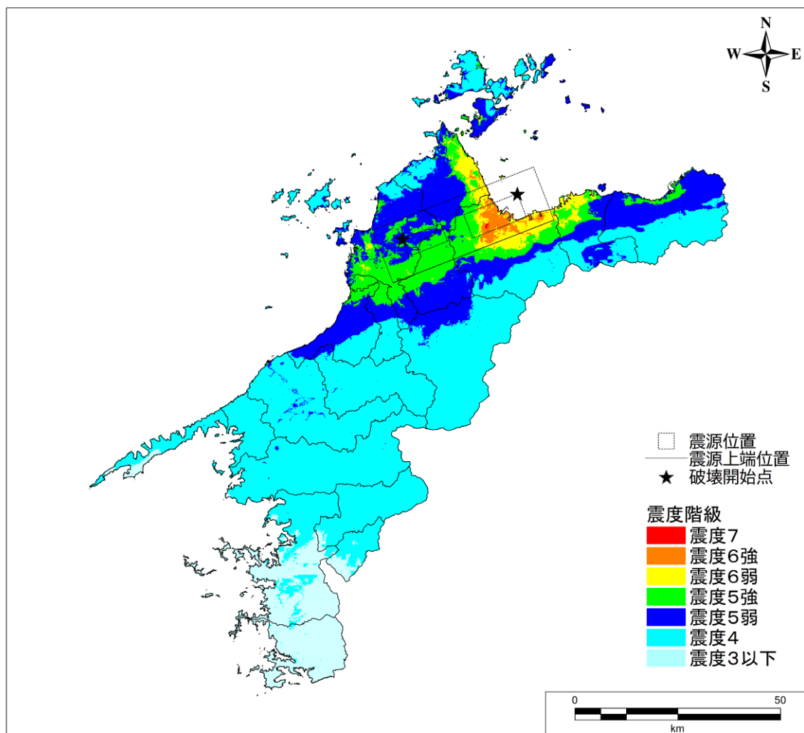
⑤中央構造線断層帯（石鎚山脈北縁西部区間）の震度分布
