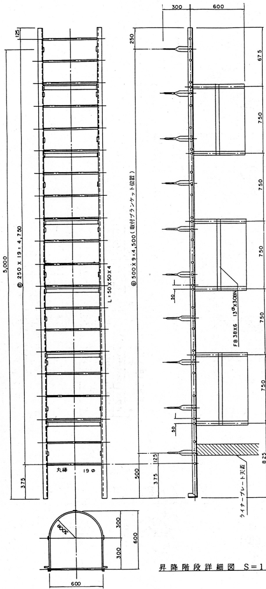
昇降階段 10m 当り材料表
