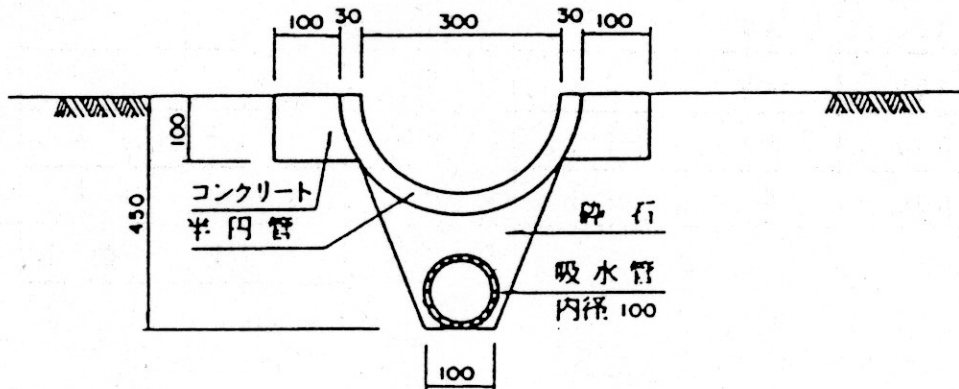
30型 半円管詳細図 S = 1:10 (mm)
