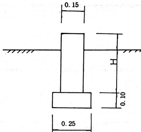
鍬止コンクリート 1m当り材料表
