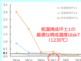
焼成温度と吸水率の関係
