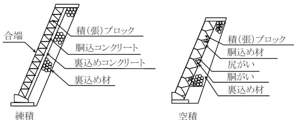
図3-2-5 コンクリートブロック工
