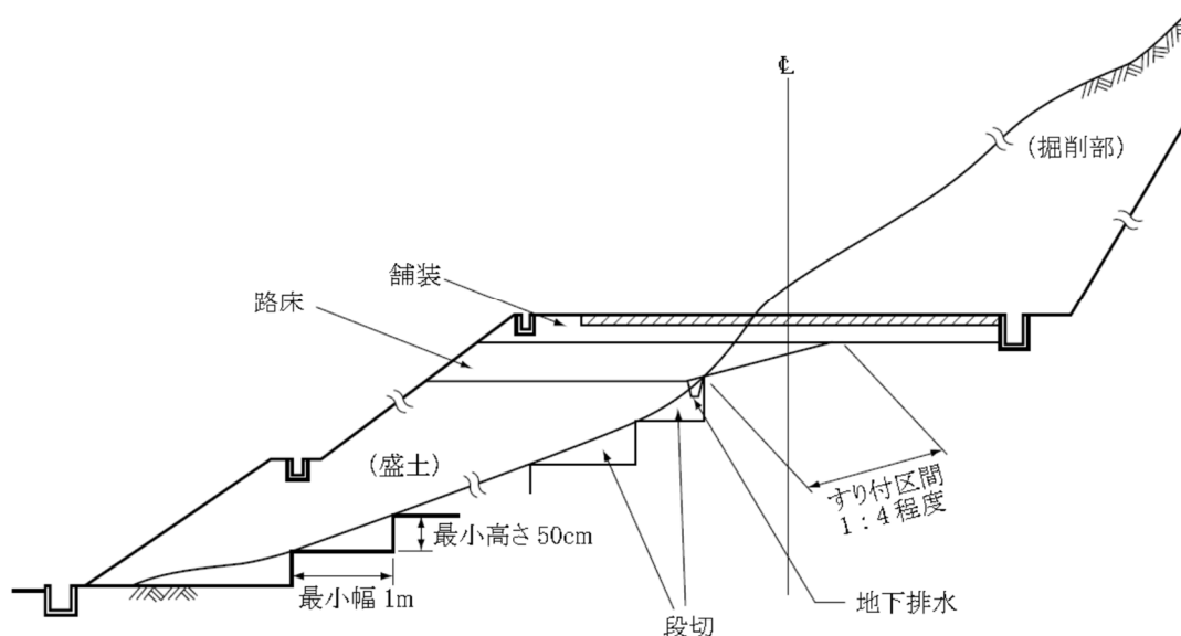
図1-2-2 盛土基礎地盤の段切
