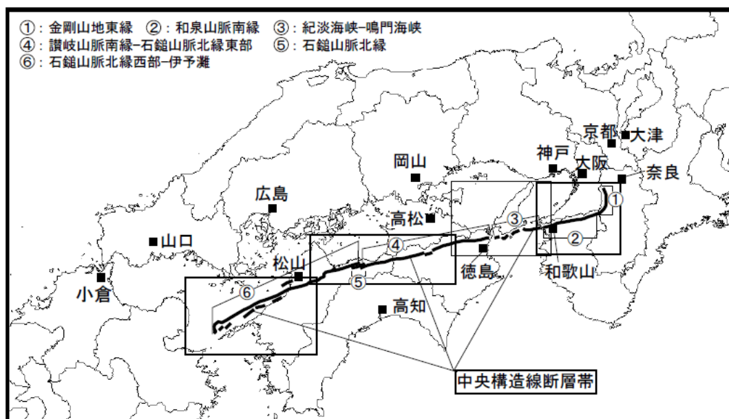
(出典：「中央構造線断層帯（金剛山地東縁－伊予灘）の評価」地震調査研究推進本部)
