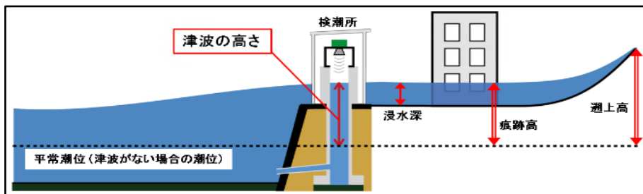
津波の高さの定義【気象庁】
