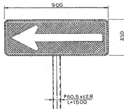
誘導標2型
