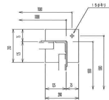
ベースプレート詳細 S=1/10
